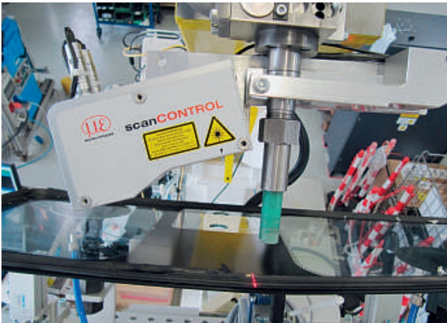
Die Laserlinie wird möglichst nah an die Düse positioniert, um eine durchgängige Messung zu gestatten
