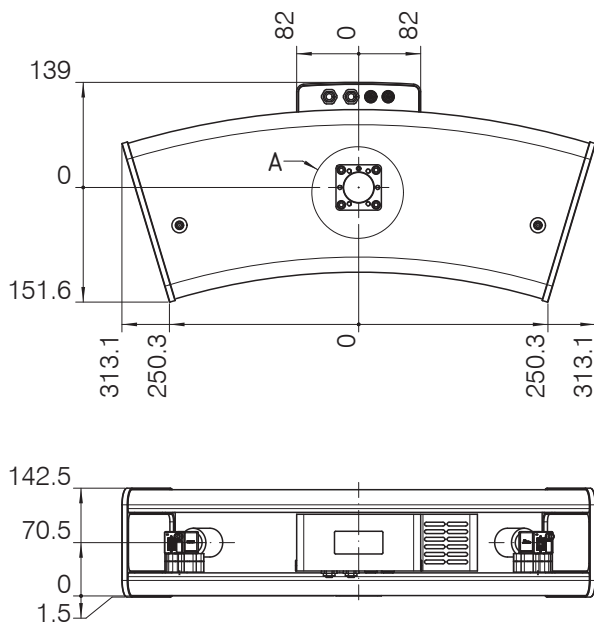
Abb. 8 Maßzeichnung Sensor surfaceCONTROL 3D SC25x0, Abmessungen in mm
