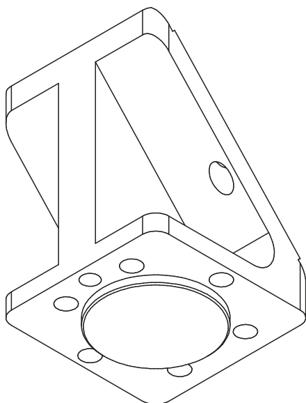
Abb. 33 Ansicht 47° Montageadapter für SC25x0 von unten (Sensorseite)
