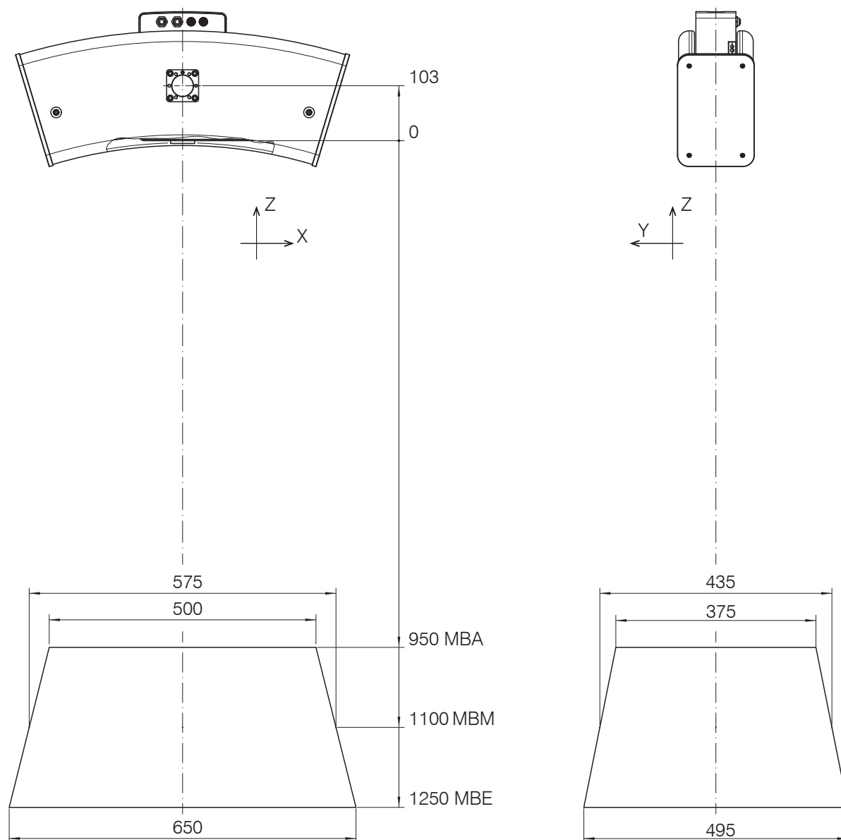
Abb. 9 Maßzeichnung Messfeld surfaceCONTROL 3D SC25x0-575, Abmessungen in mm
