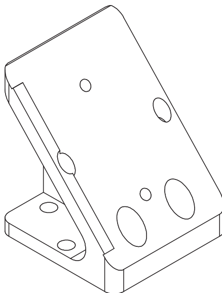
Abb. 34 Ansicht 47° Montageadapter für SC25x0 von oben (Stativseite)
