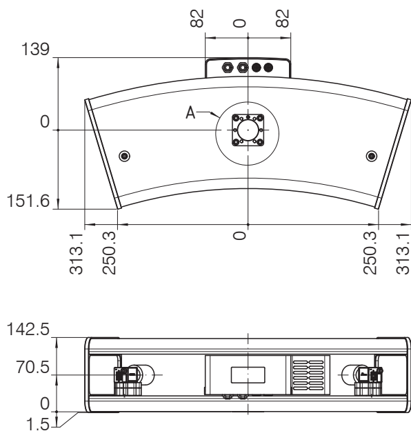
Abb. 6 Maßzeichnung Sensor surfaceCONTROL 3D SC25x0, Abmessungen in mm
