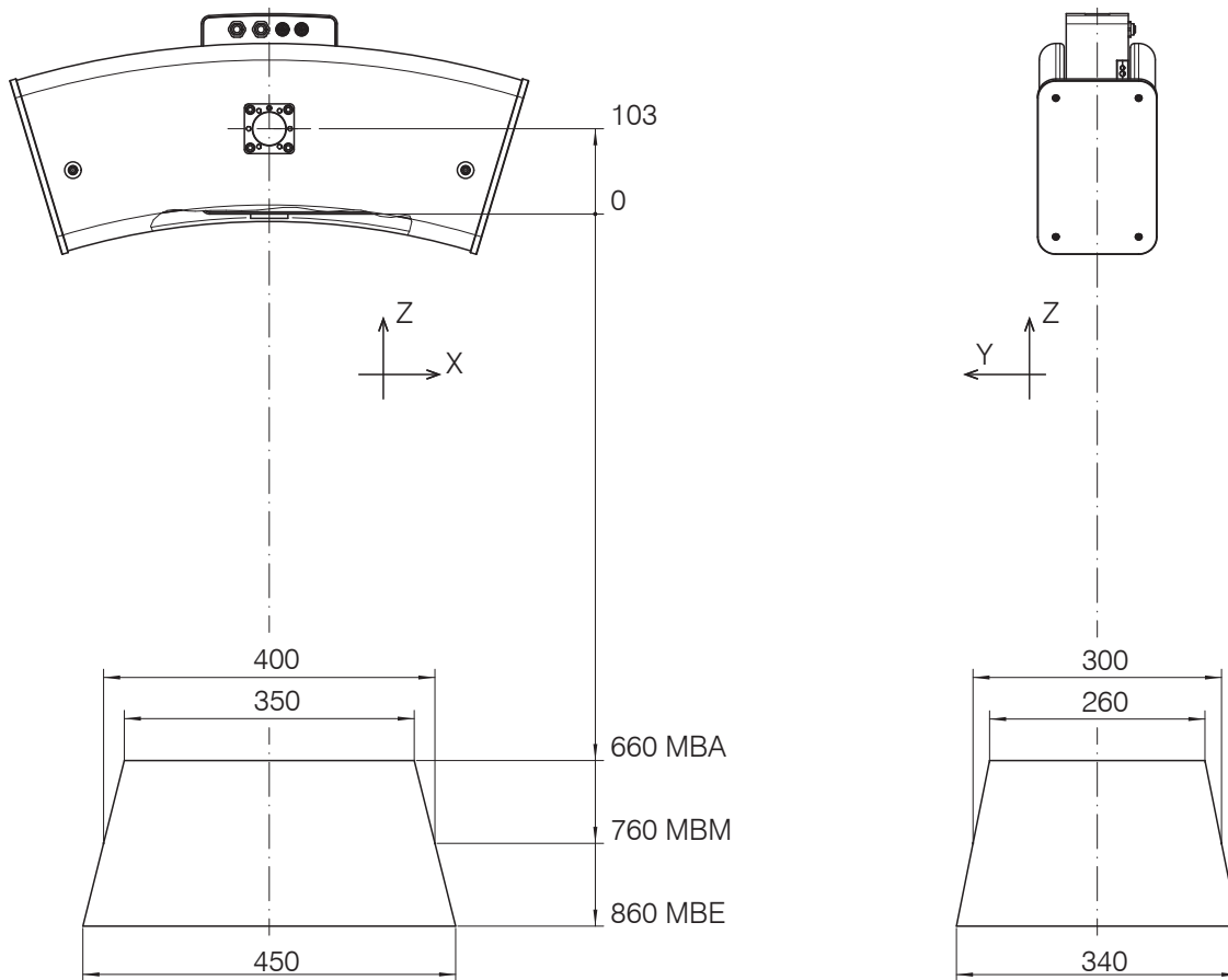
Abb. 7 Maßzeichnung Messfeld surfaceCONTROL 3D SC25x0-400, Abmessungen in mm
