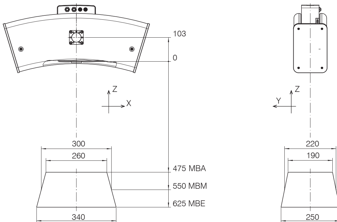
Abb. 5 Maßzeichnung Messfeld surfaceCONTROL 3D SC25x0-300, Abmessungen in mm
