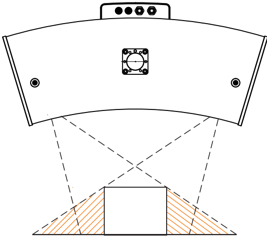
Abb. 30 Abschattung Empfänger
