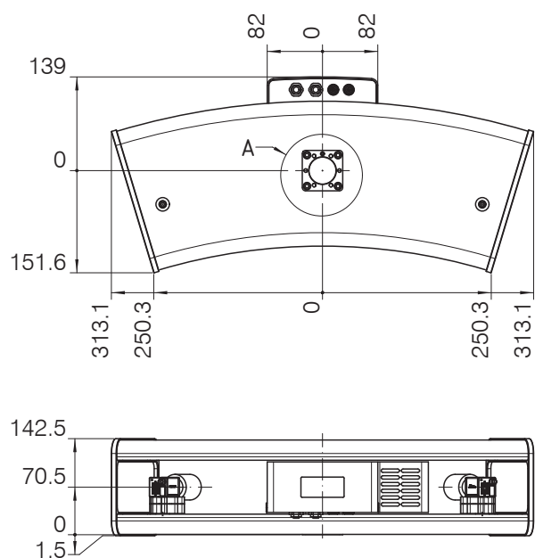
Abb. 10 Maßzeichnung Sensor surfaceCONTROL 3D SC25x0, Abmessungen in mm
