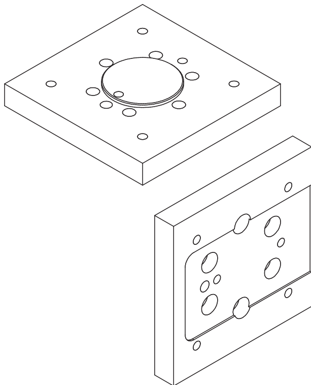
Abb. 32 Ansicht Montageadapter für SC25x0
