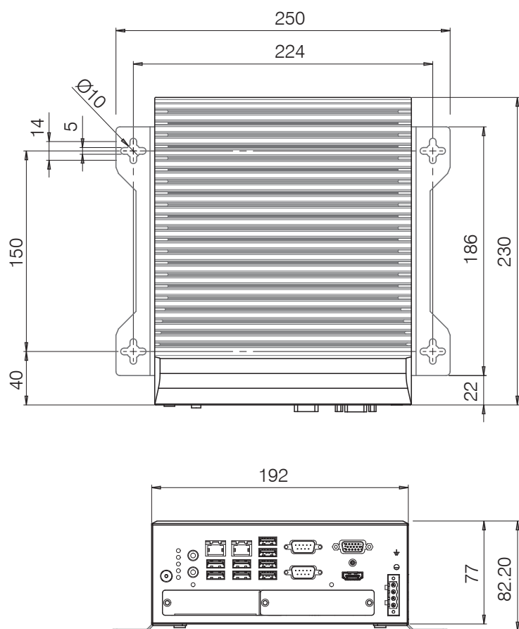
Abb. 12 Maßzeichnung Controller SC2500 mit Montageadapter, Abmessungen in mm
