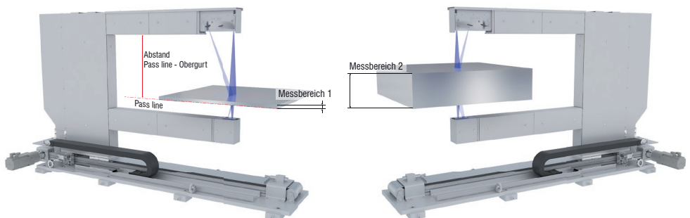
Sequentielle Messbereiche für große Dickenvariation
