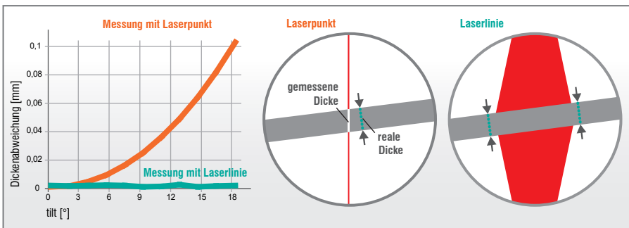
Beispielhafte Abweichung des Dickenwertes bei Bandverkippen bei 4 mm Materialdicke
