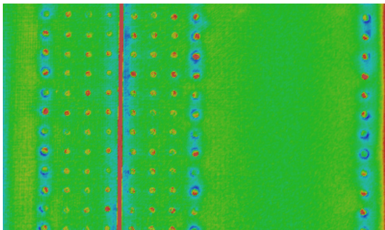
Nietprüfung: Verformung, Höhe und Position des Nieten
