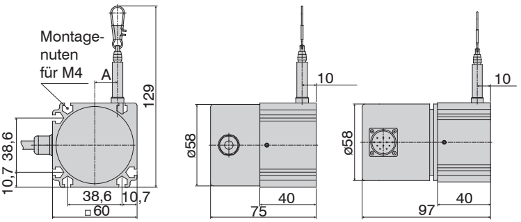
Maßzeichnung WDS- ... - P60 - XX - XXX Maßzeichnung WDS- ... - P60 - CR - HTL/TTL Maßzeichnung WDS- ... - P60 - SR - SSI
