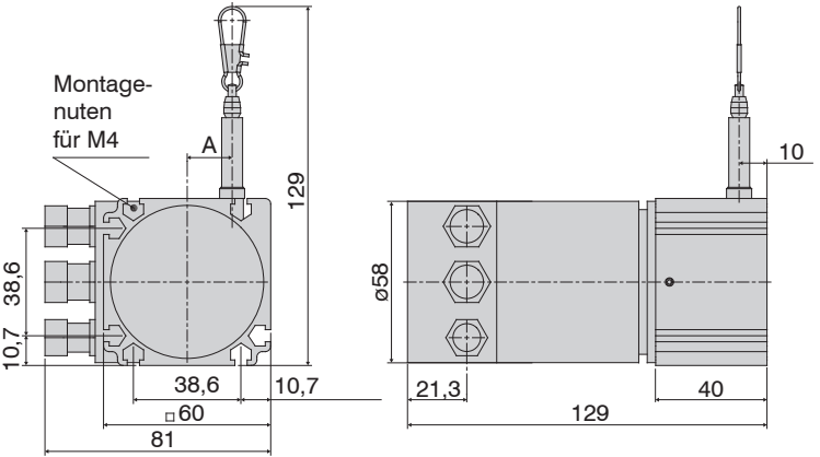
Maßzeichnung WDS- ... - P60 - BH - CO/PB/PN/ENIP/CAT, Abmessungen in mm
