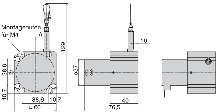
Maßzeichnung WDS- ... - P60 - CR - P, Abmessungen in mm
