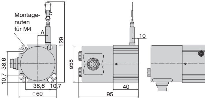
Maßzeichnung WDS- ... - P60 - SR - U/I, Abmessungen in mm
