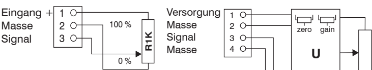
Ausführung mit Potentiometerausgang
